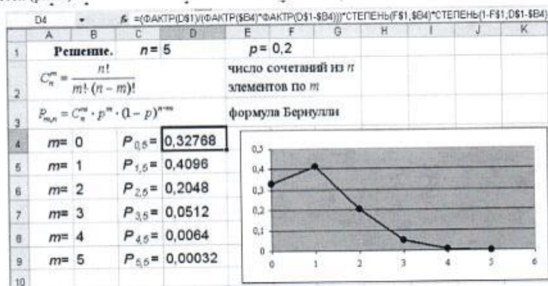
Рисунок 1 - Применение формулы Бернулли
